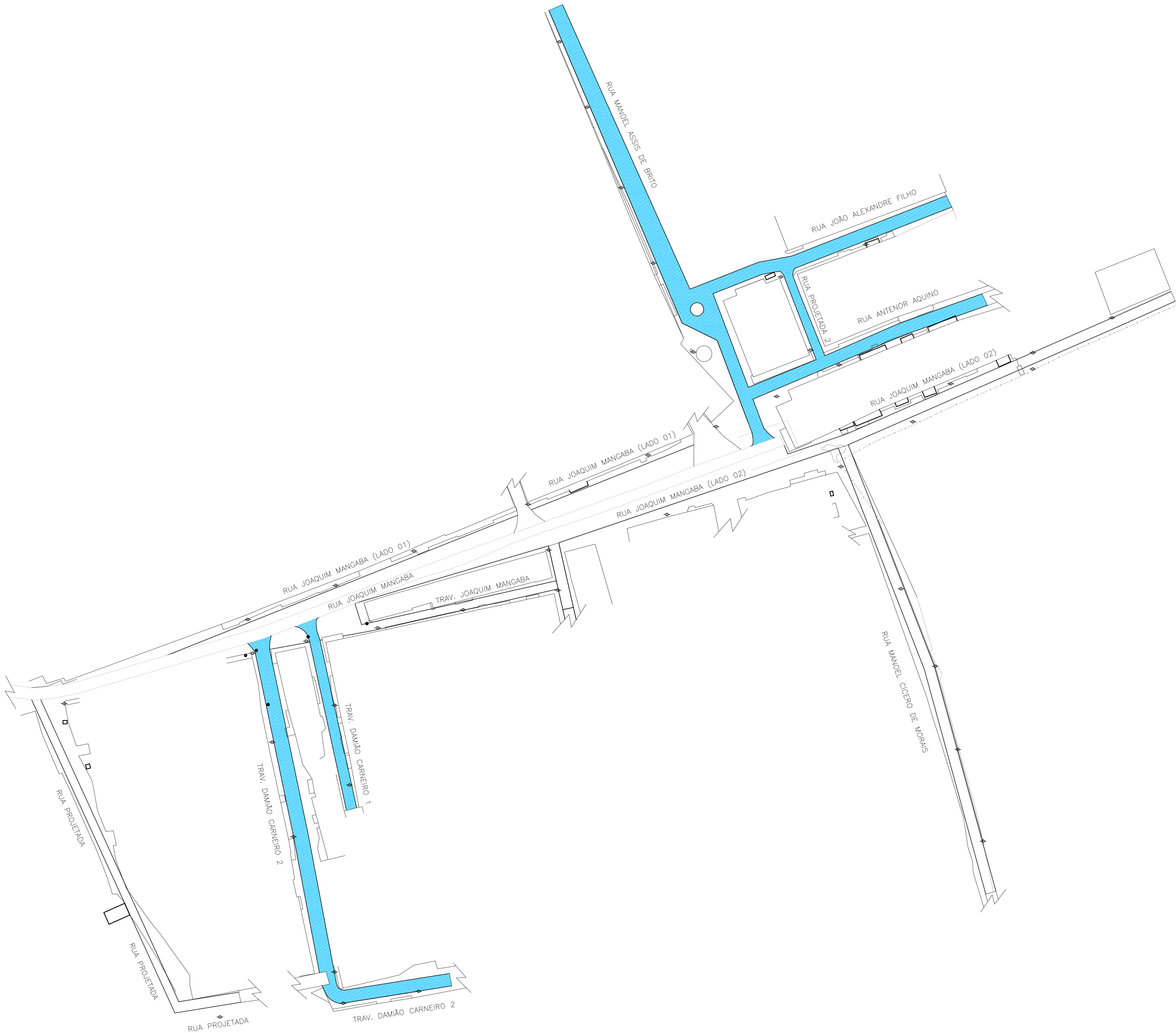
PLANTA DE SITUAÇÃO Pavimentações, Jucurutu/RN Escala: 1/1000
