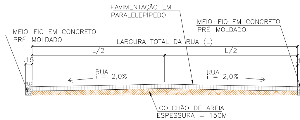
CORTE TRANSVERSAL - TRECHO 13 Pavimentações, Jucurutu/RN Sem escala
