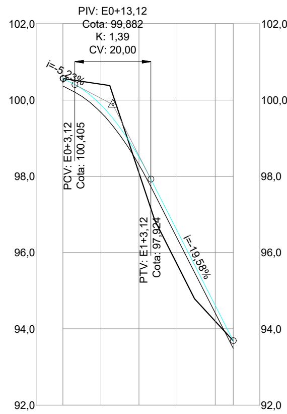
TRECHO 13-SERRA DO JOÃO DO VALE - E00 ATÉ E02+4,75m PERFIL LONGITUDINAL - ESC.: V=1:100 H=1:1000
