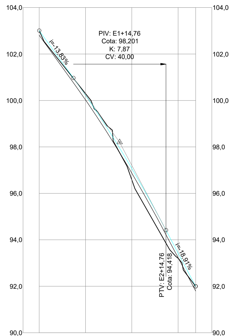
TRECHO 17 - SERRA DO JOÃO DO VALE - E0+0 ATÉ E3+7,57 PERFIL LONGITUDINAL - ESC.: V=1:100 H=1:1000
