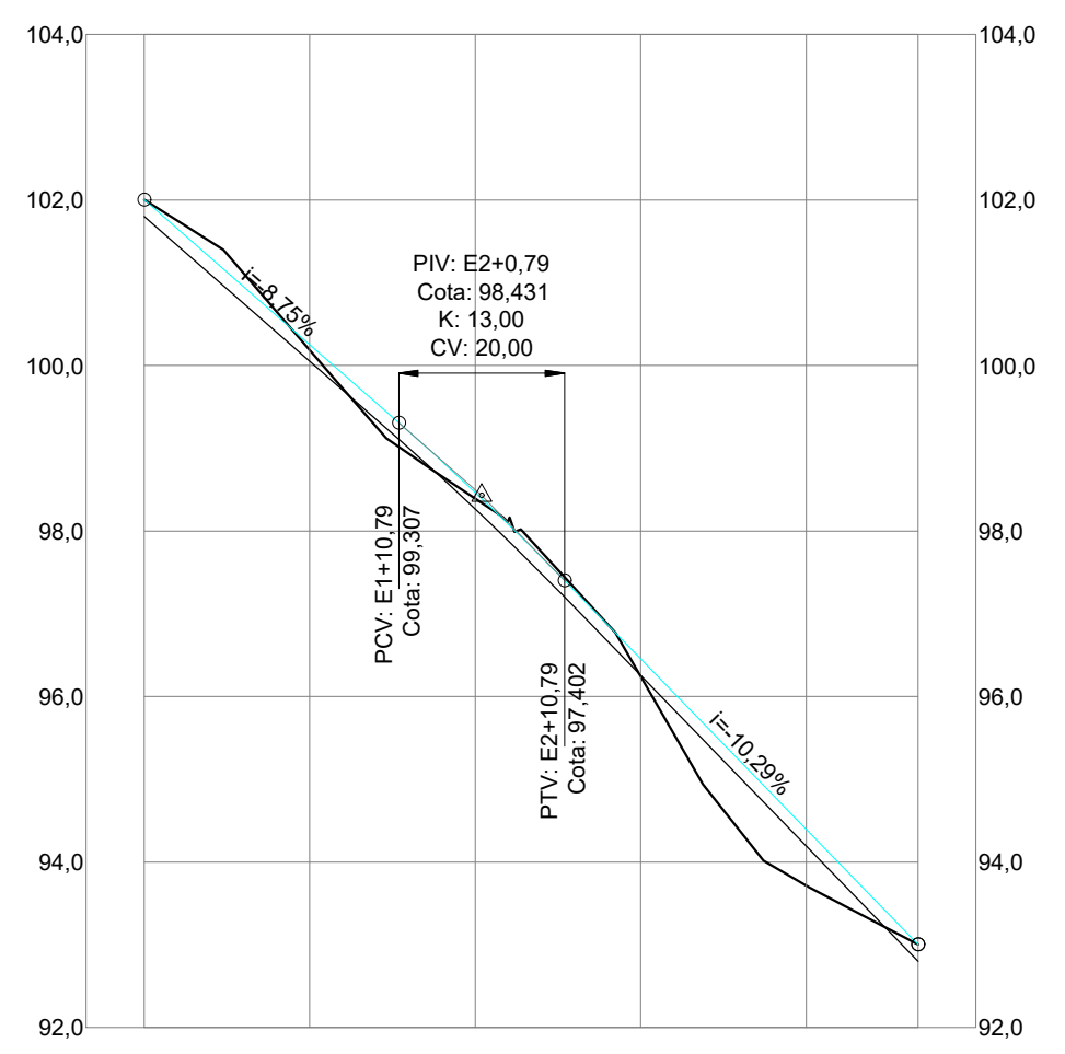
TRECHO 07-SERRA JOÃO DO VALE - E00 ATÉ E04+13,52m PERFIL LONGITUDINAL - ESC.: V=1:100 H=1:1000
