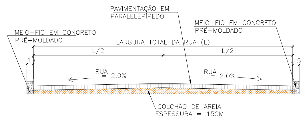
CORTE TRANSVERSAL - TRECHO 07 Pavimentações, Jucurutu/RN Sem escala
