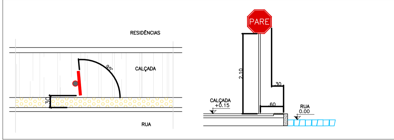
DETALHE DA PLACA "PARE" Jucurutu/ RN Escala: 1/50
