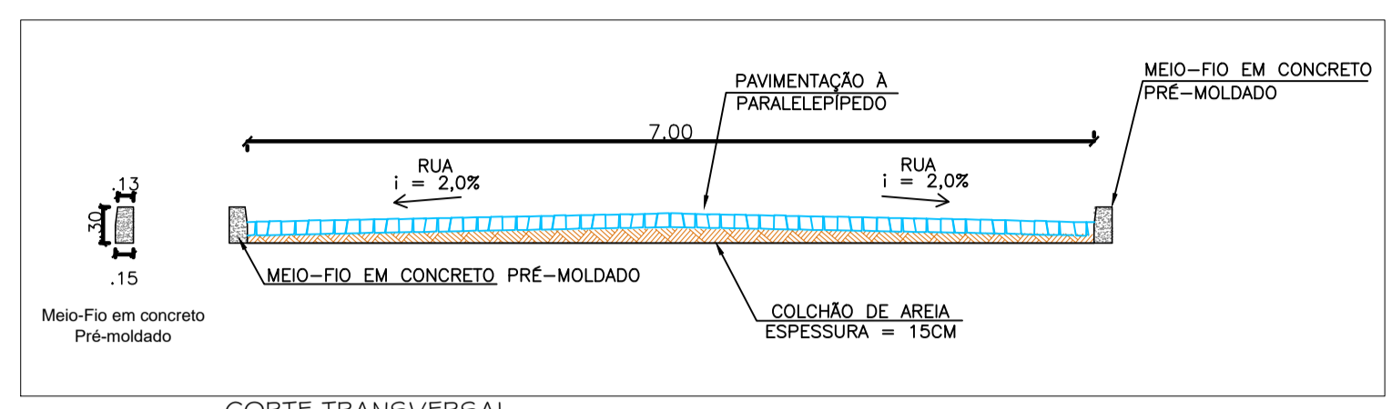
CORTE TRANSVERSAL Jucurutu/ RN Escala: 1/50
