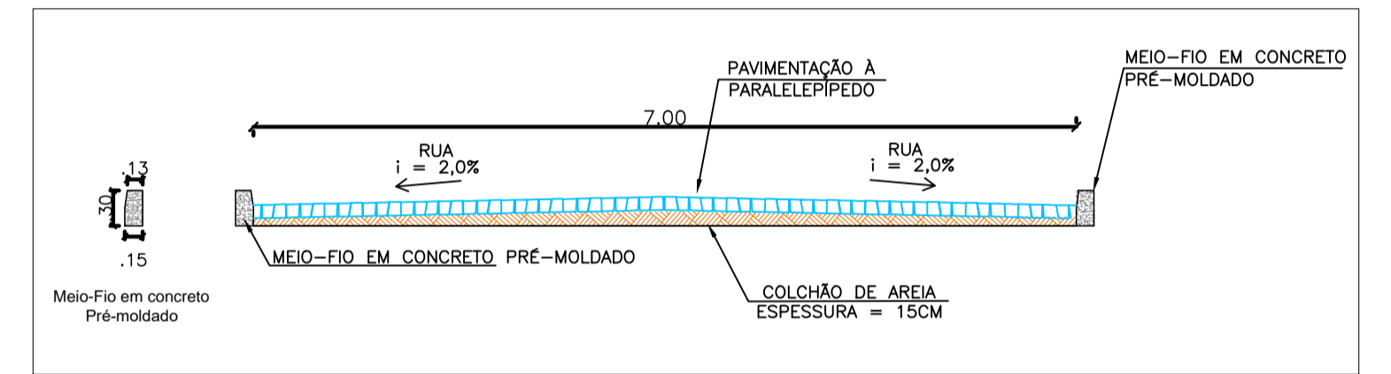
CORTE TRANSVERSAL Jucurutu/ RN Escala: 1/50
